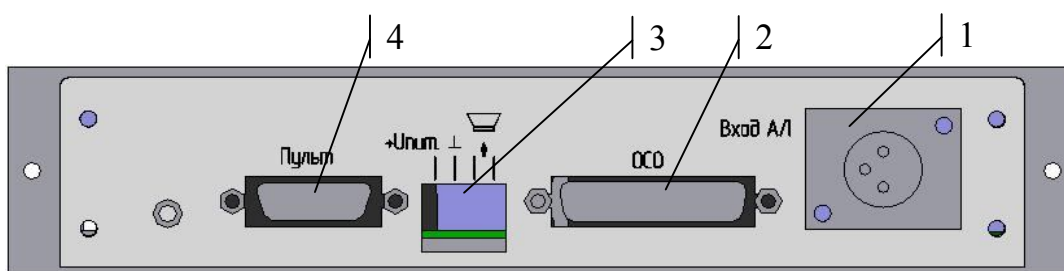
Рисунок 8 - Внешний вид правой панели ДК-ОСО-1 в исполнении для монтажа в 19” стойку
