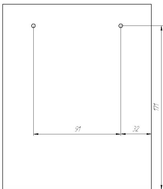
Рисунок 15 – Установочные размеры для крепежа ДК-ОСО-1
