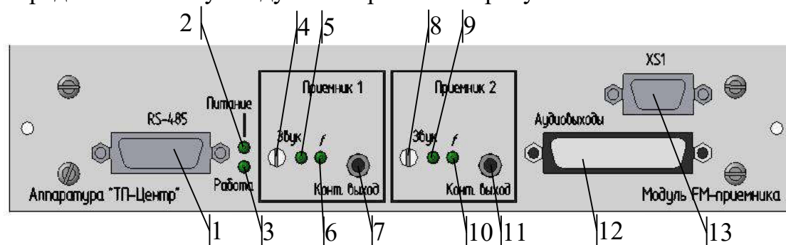
Рисунок 3 – Расположение элементов коммутации и индикации на передней панели субмодуля FM-приемника
