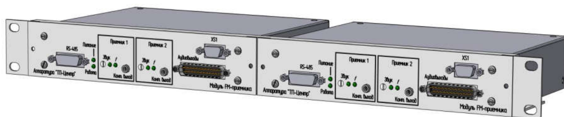
Рисунок 1 – Четырехканальный модуль FM-приемника
