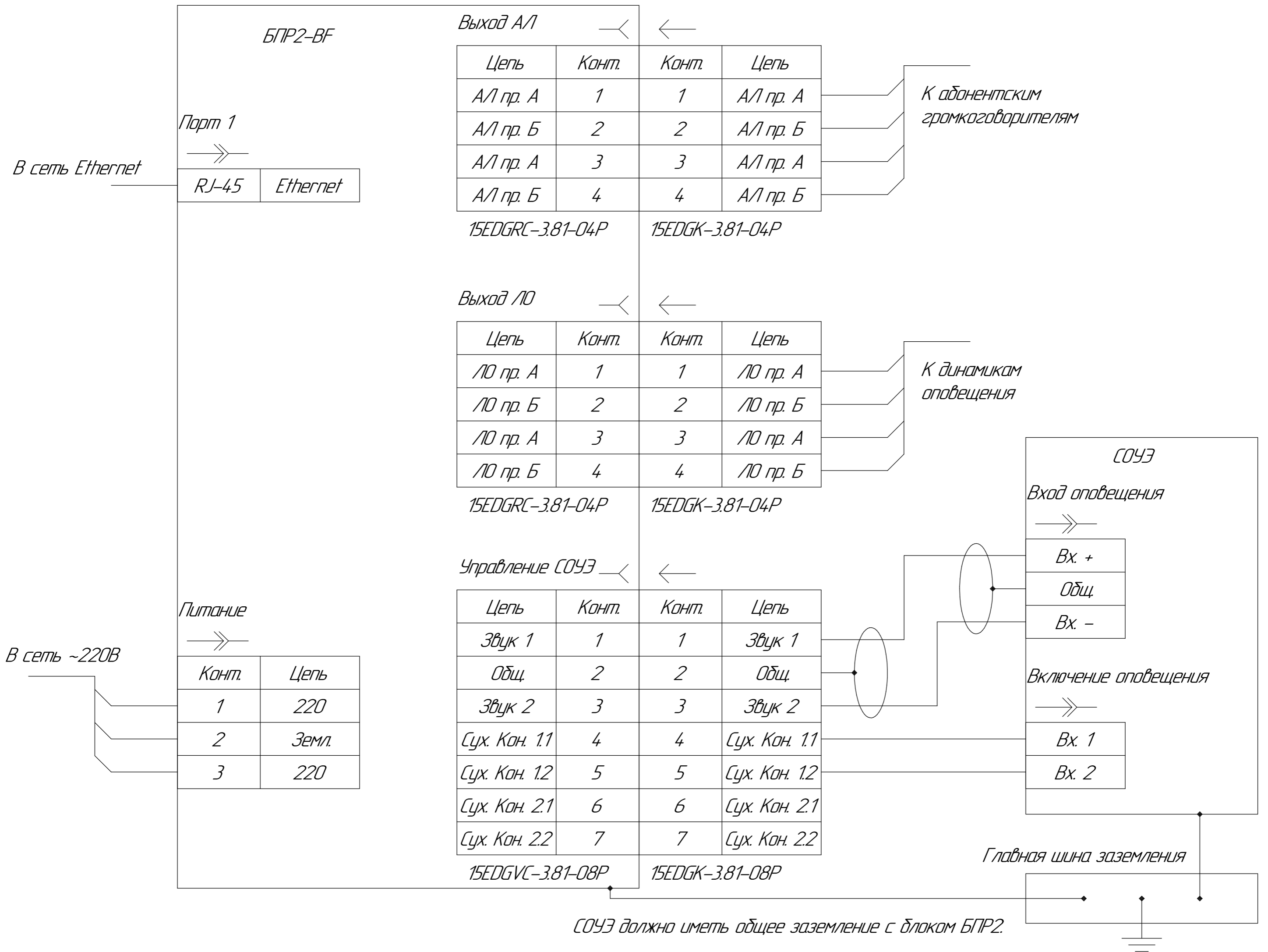
Схема сопряжения БПР2-ВФ и одной СОУЭ с симметричным входом.
