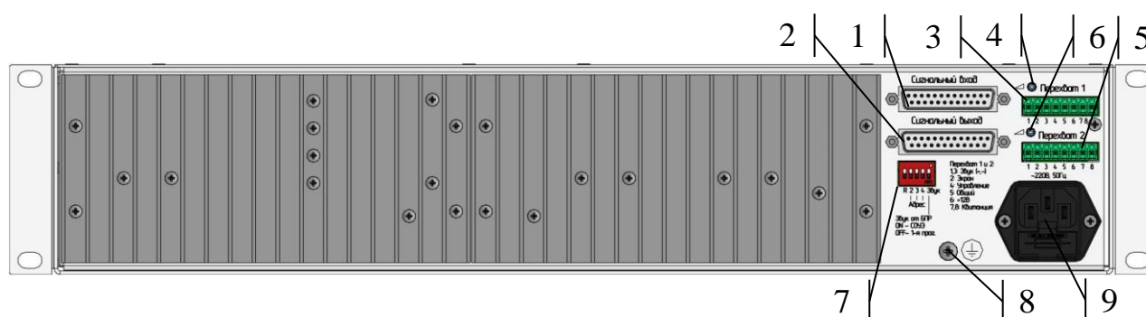
Рисунок 4 – Элементы задней панели
