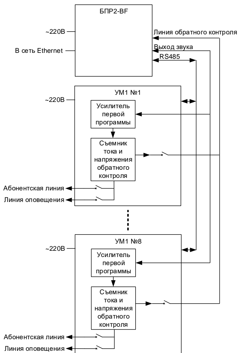
Рисунок 5 – Структурная схема соединения УМ1 и блока БПР2-ВФ
