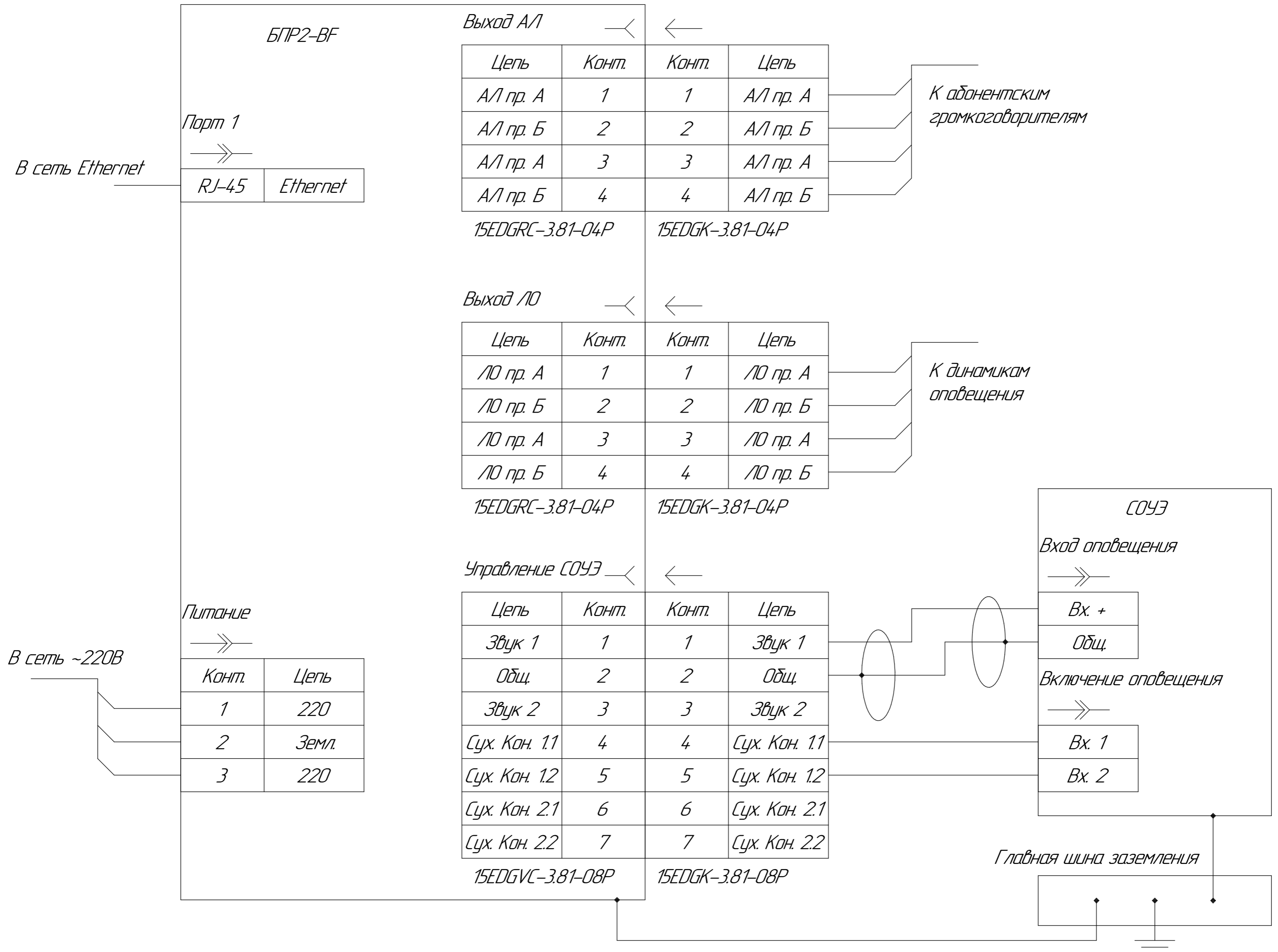
Схема сопряжения БПР2-ВФ и одной СОУЭ с несимметричным звуковым входом.
