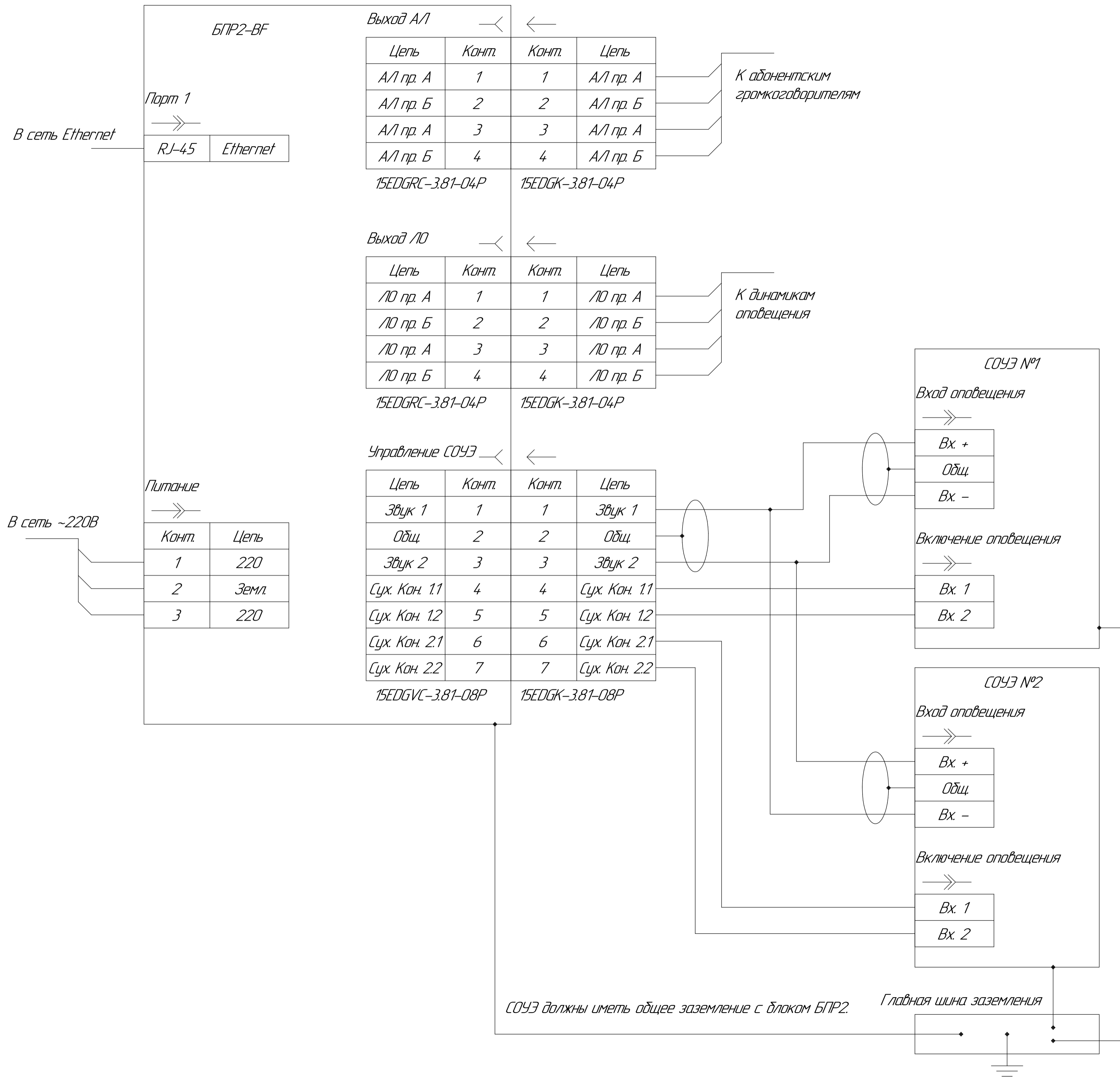
Схема сопряжения БПР2-ВФ и двух СОУЗ
